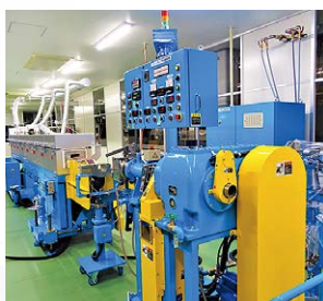
シリコンゴム押出機
